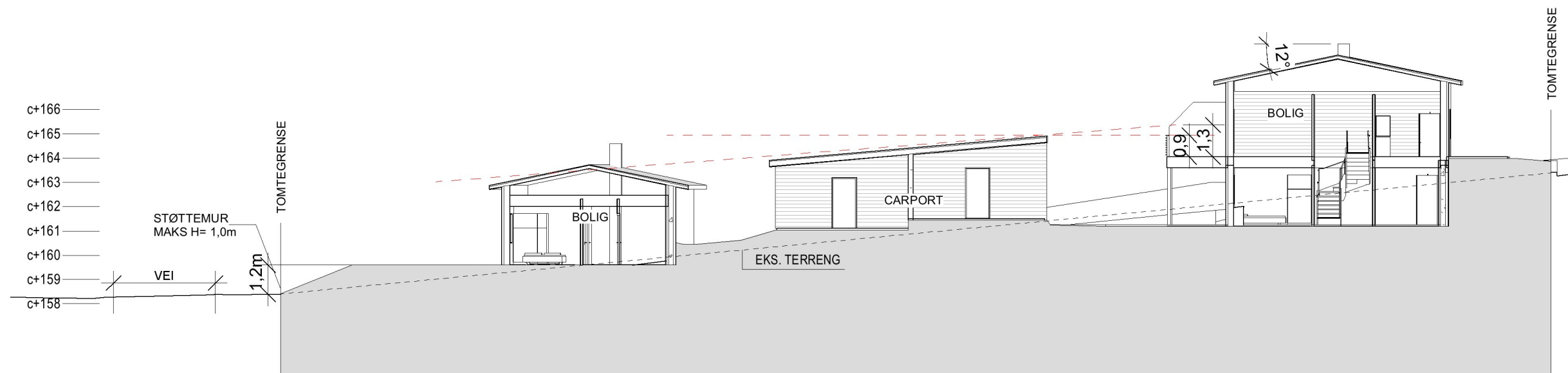
Terrengsnitt 1-1 1 : 200
