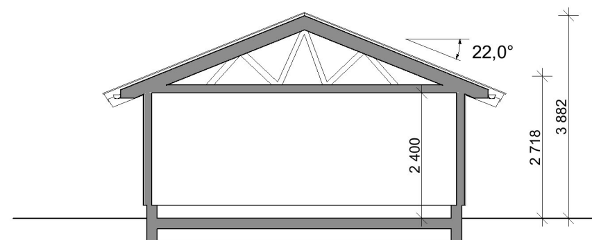
1:100 S-B
