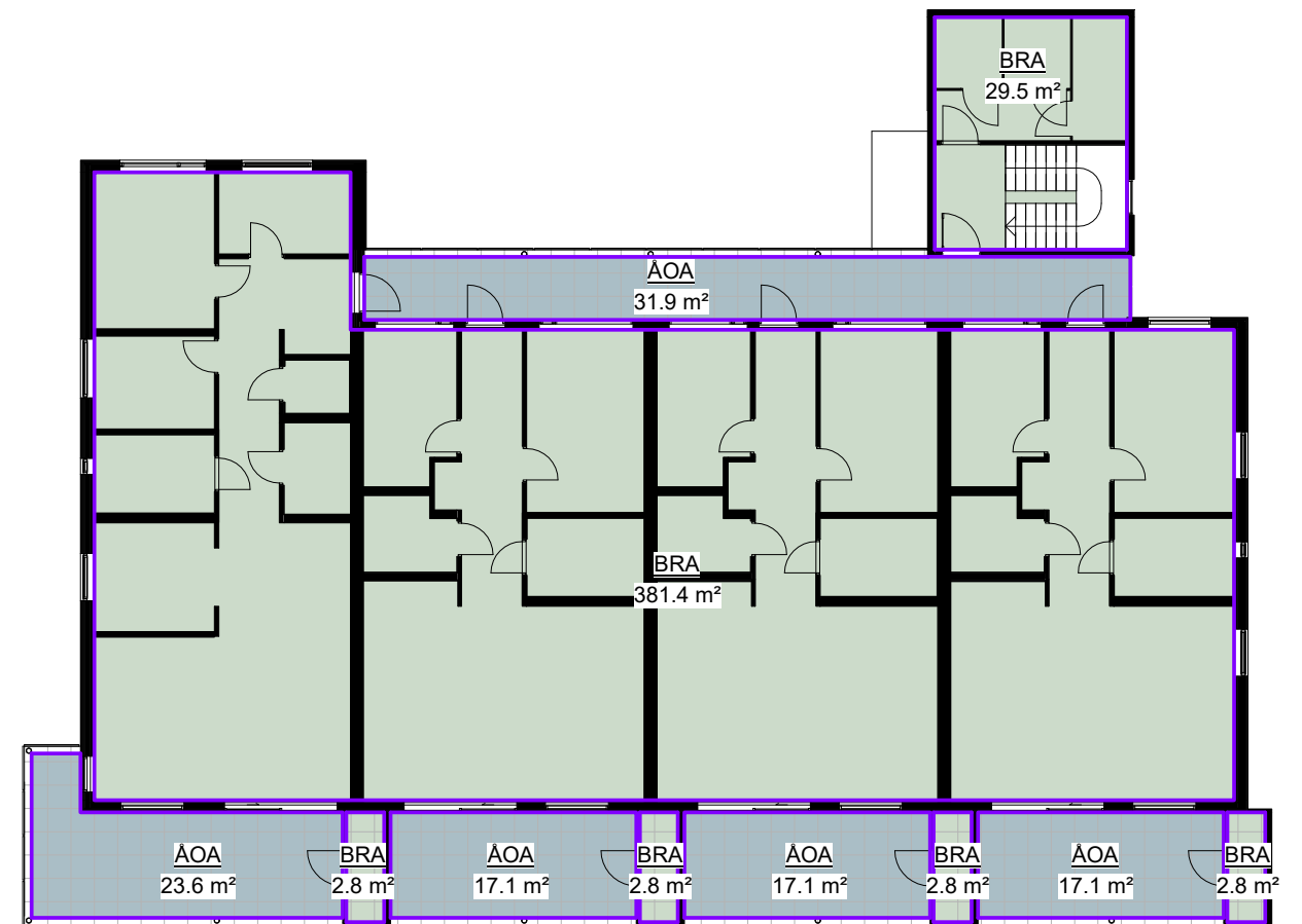
2 Plan 2 - B 1 : 200
