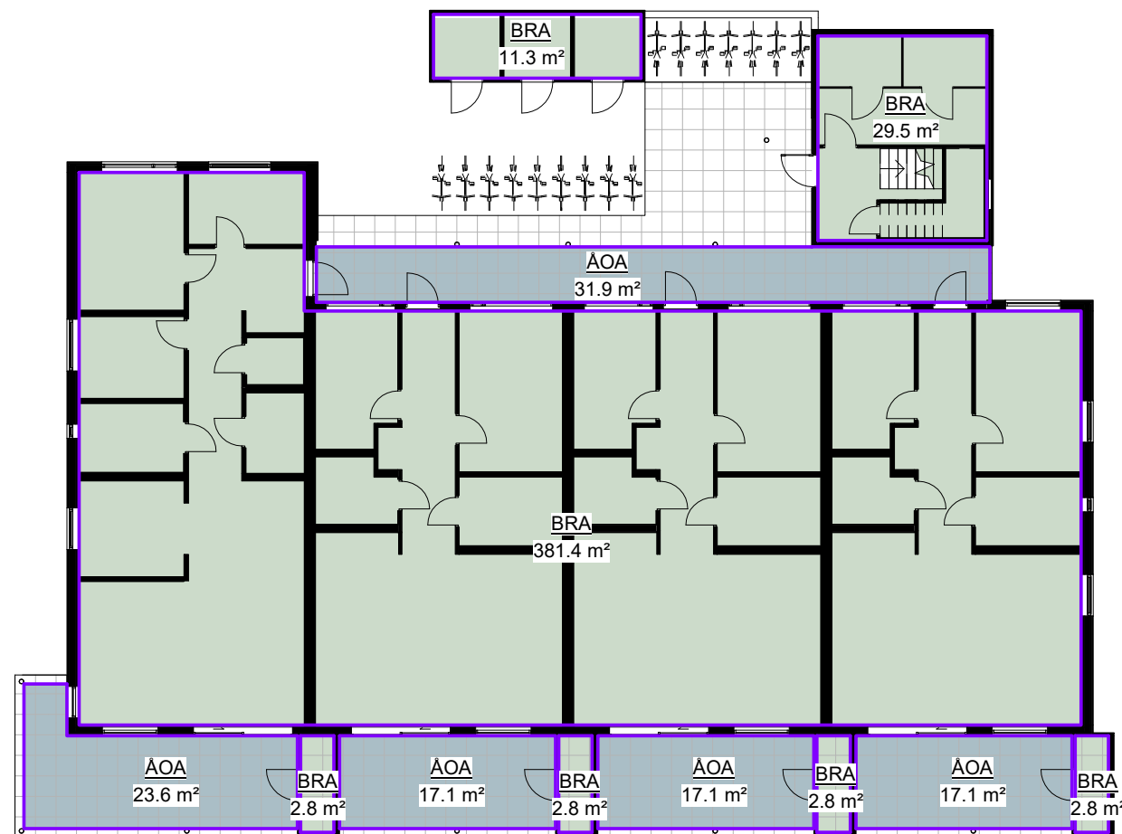
1 Plan 1 - B 1 : 200
