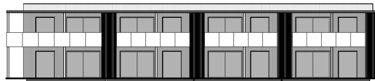
2 Fasade vest Blokk B 1 : 200
