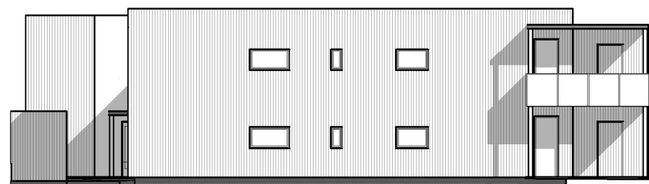
1 Fasade nord Blokk B 1 : 200
