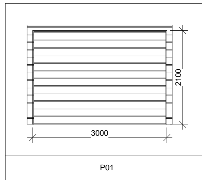
PORT 1 : 50
